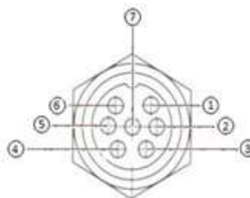
Conector 2 (fêmea)
