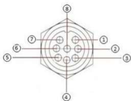
Conector 1 (fêmea)
