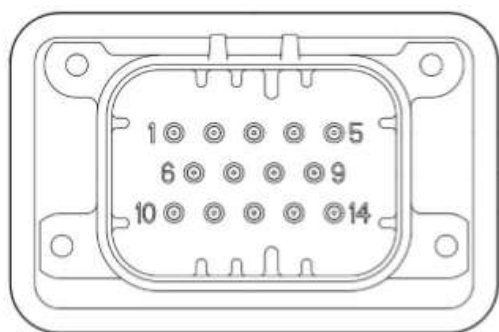
Figura 2: conector IDM-6
