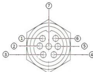
CON 2 (Pinout)
